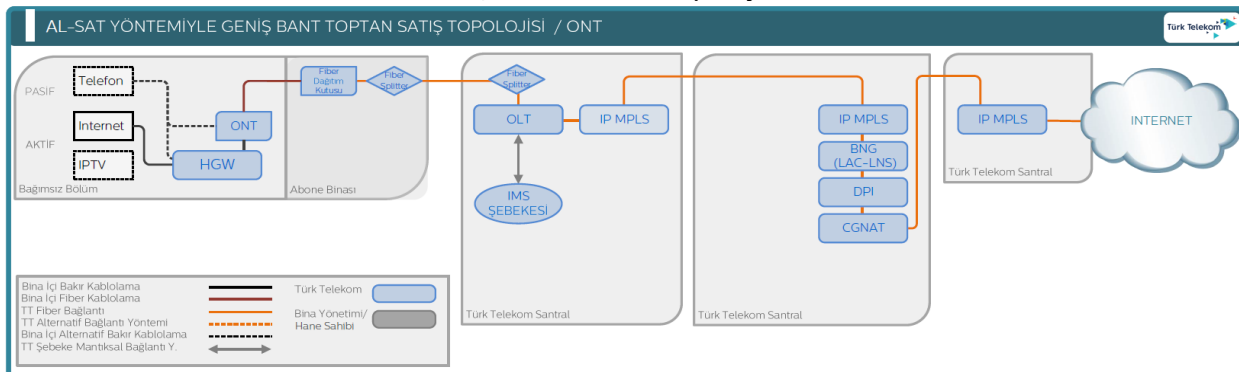
Şekil-4: PON Topolojisi
